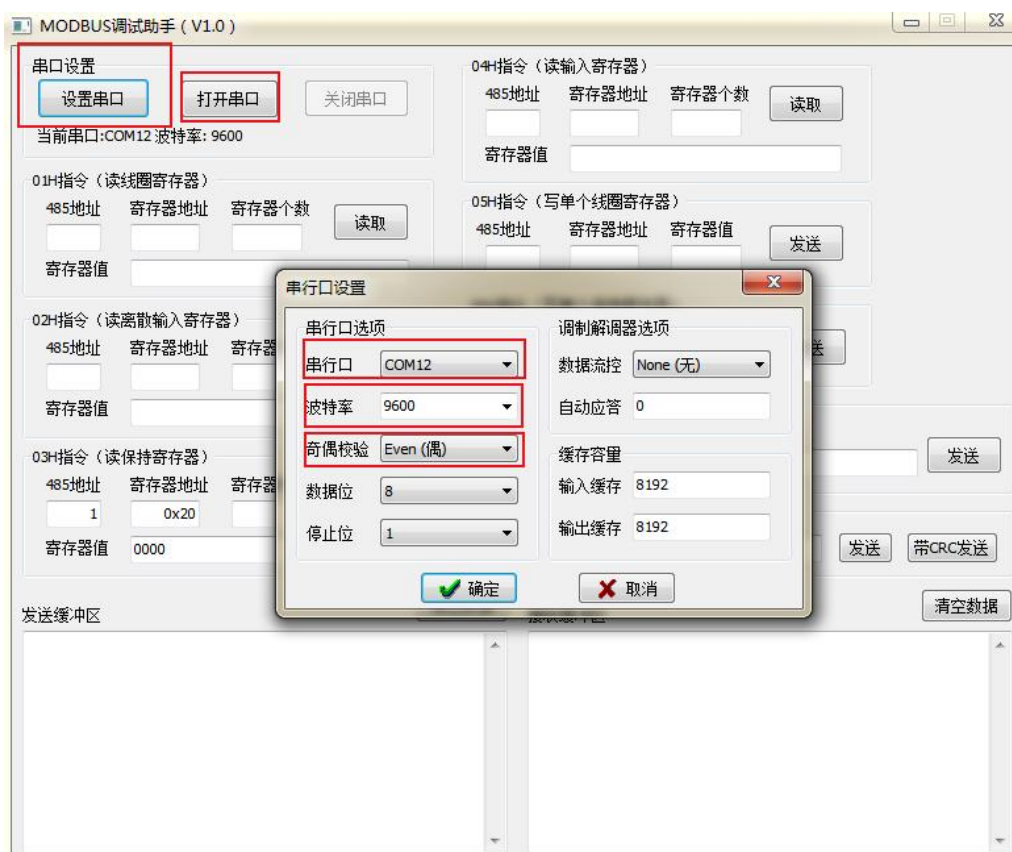
Modbus 调试助手软件连接示意图
