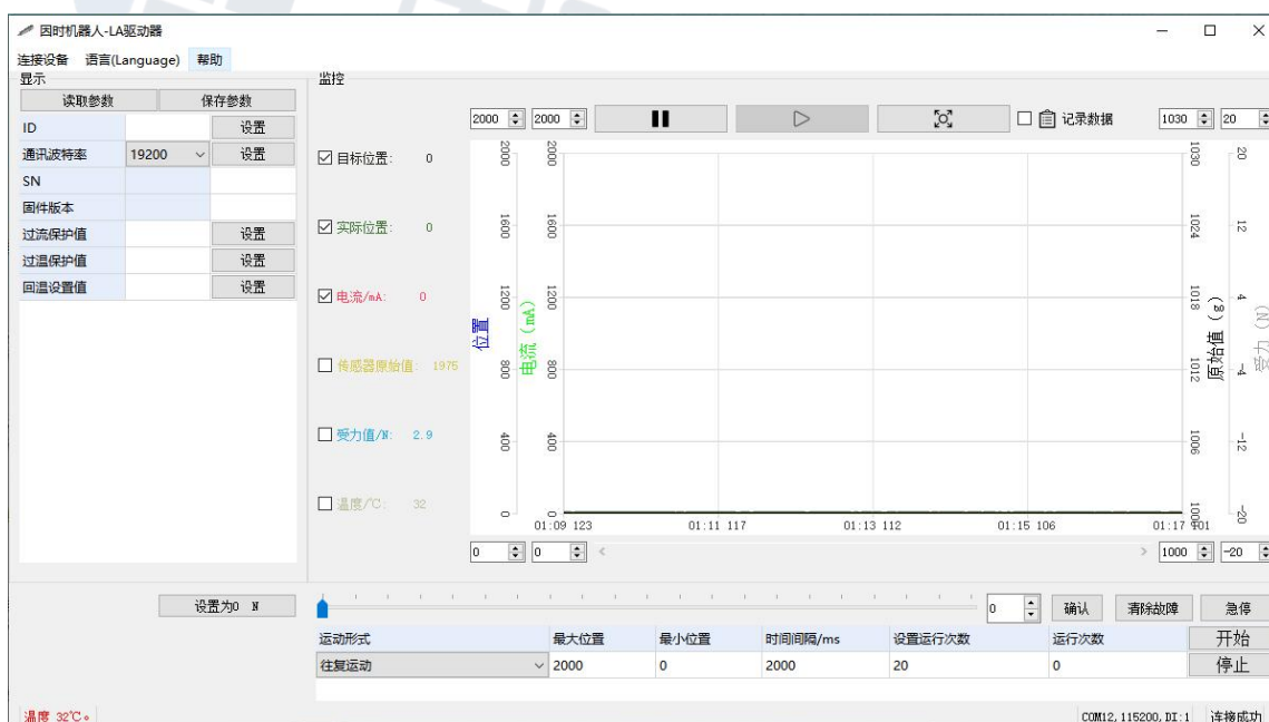
上位机软件修改波特率①
