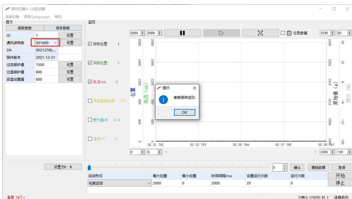
上位机软件修改波特率②
