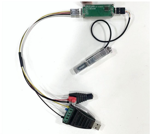
Modbus 转换器、测试线缆、电缸连接示意图
