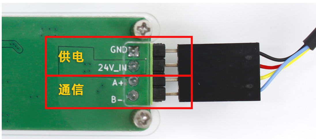
PLC 端正确接法示意图
